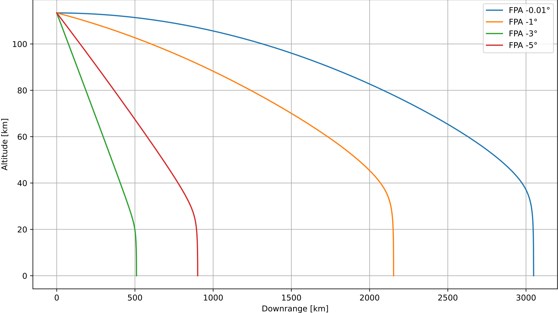
Altitude vs Downrange pour différents Flight Path Angles for a sphere of 20cm diameter and 50kg in AA7075
